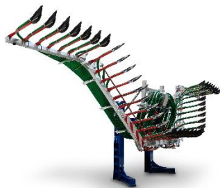
Bild 3: UniSpread im Klappvorgang: Das Universalgestänge ist ab sofort mit einer Arbeitsbreite von 10,5 Metern erhältlich.
