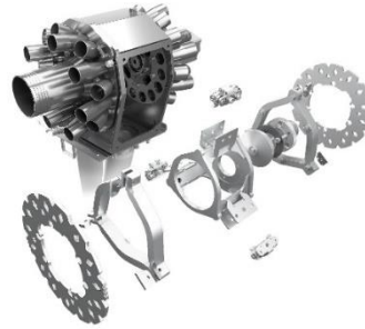
Bild 2: Premiere am Markt: Der Vogelsang-Exaktverteiler ExaCut ECC kommt ohne Luftnachsaugung aus.
