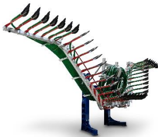
Afbeelding 3: UniSpread tijdens het uitklapproces: De universele bemester is nu verkrijgbaar met een werkbreedte van 10,5 meter.
